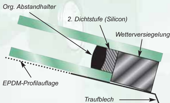
Abb. 3 Fehlerhafte Traufpunktversiegelung
